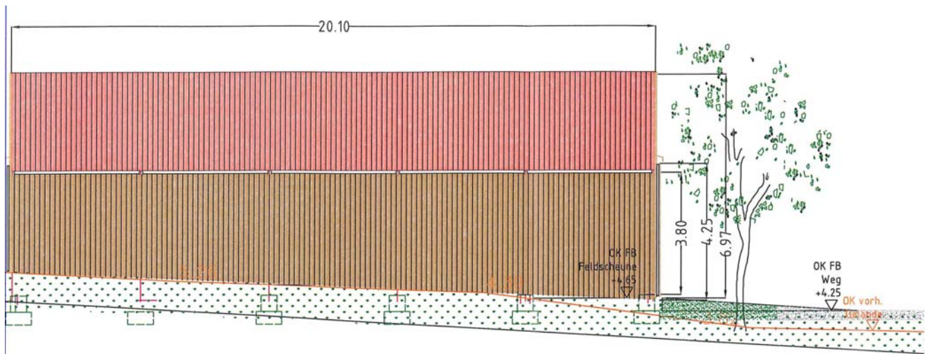
Ansicht Süd - Ost
