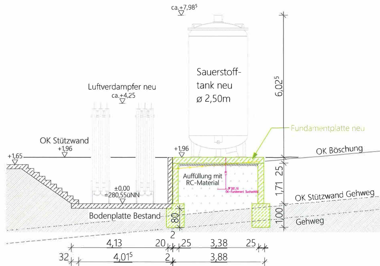
Schnitt C-C M 1:100
