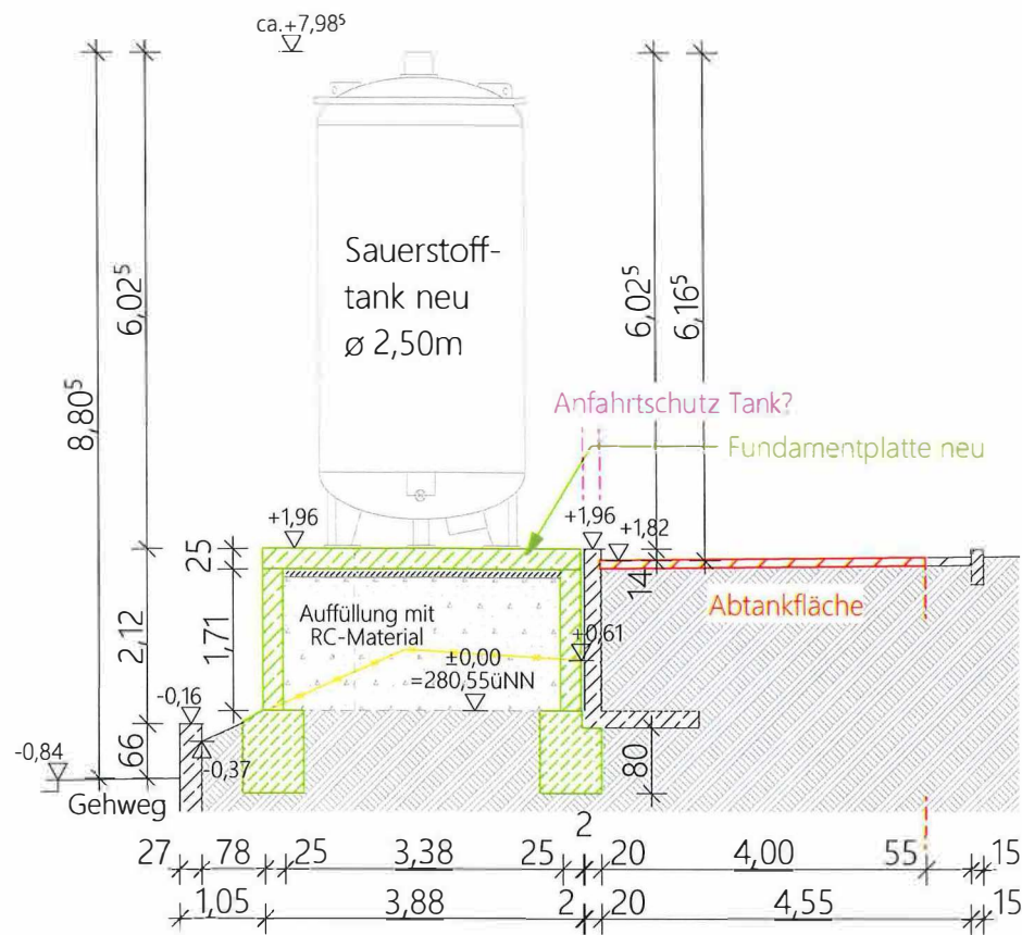
Schnitt A-A M 1:100
