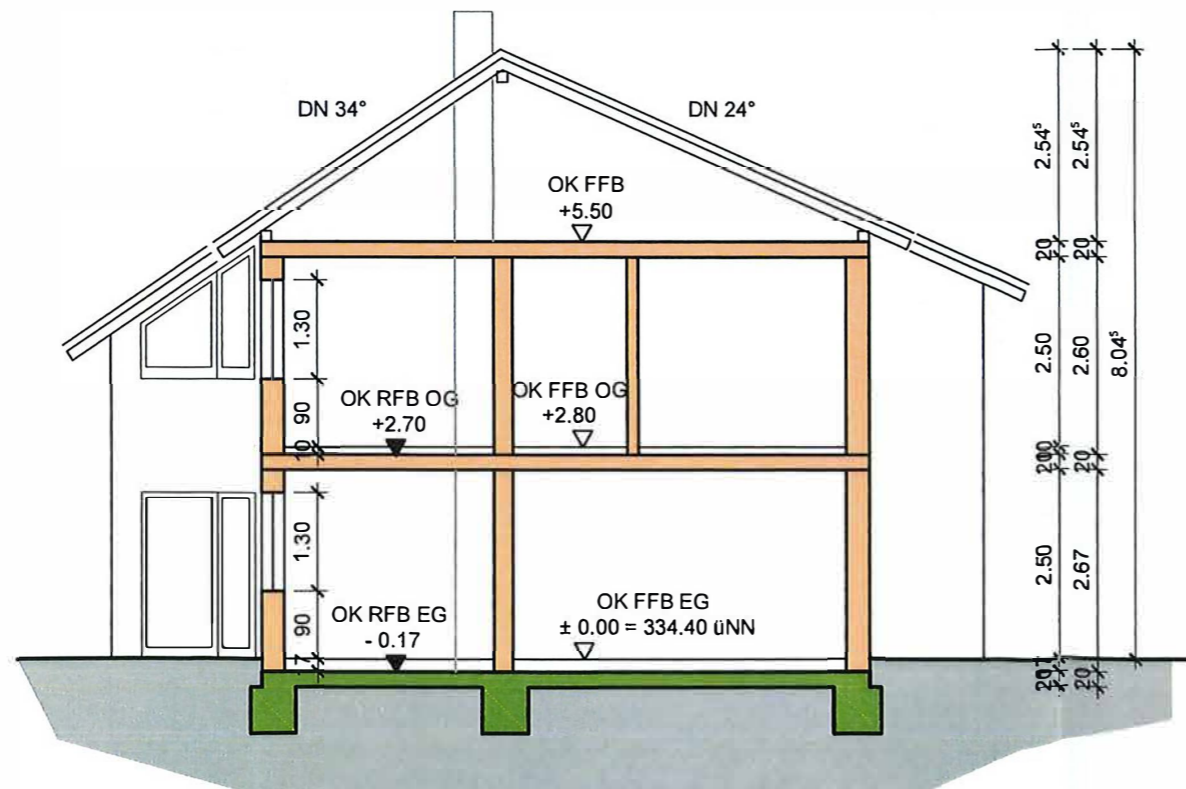
Schnitt
