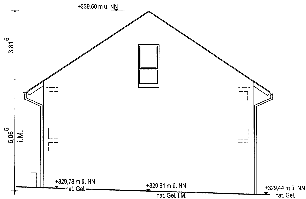
NORDOSTSEITE (GIEBELSEITE)
