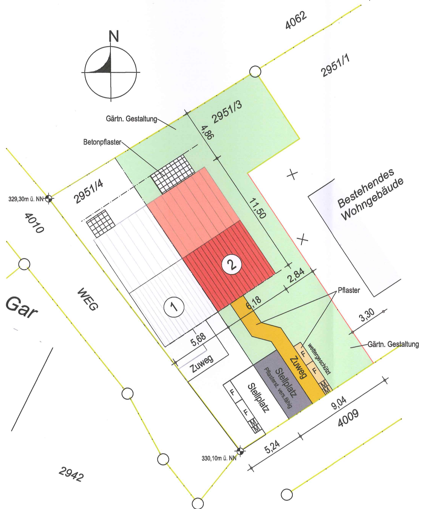
FREIFLÄCHEN-GESTALTUNGSPLAN M 1 : 200
